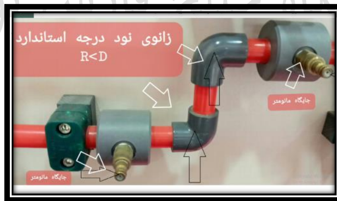
شکل (۷): خم نود درجه با گوشه استاندارد
