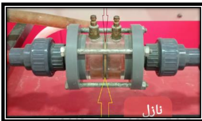
شکل (۱۰) : نازل
